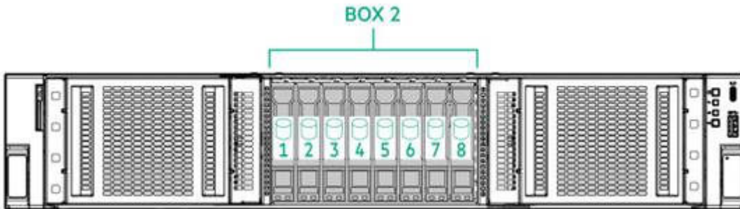
36EDSFF drive bay, SFF/EDSFF CTO server (P81948-B21)
